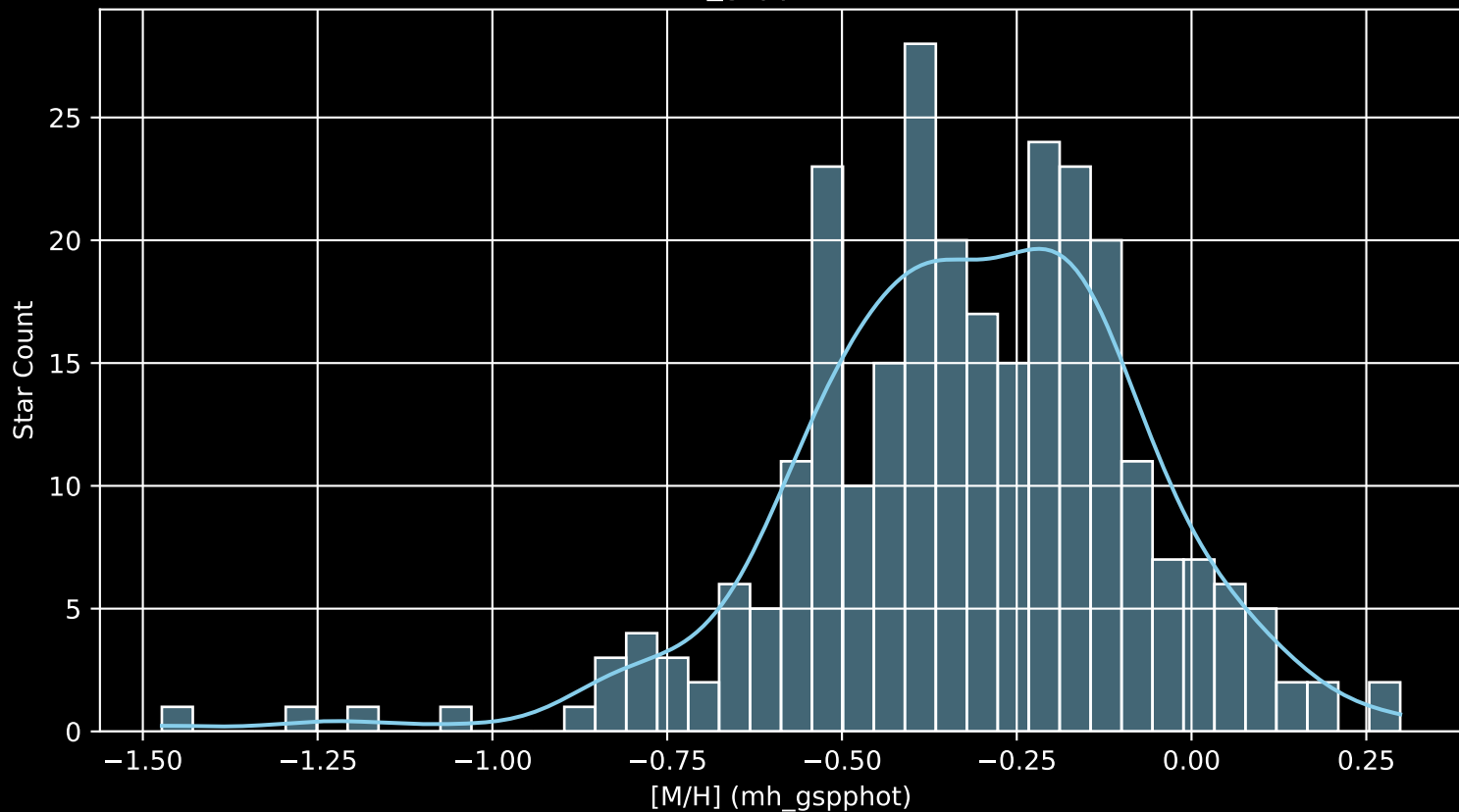
GALAH DR4 Field: [2547] [M/H] (mh_gspphot) (n= 276)
