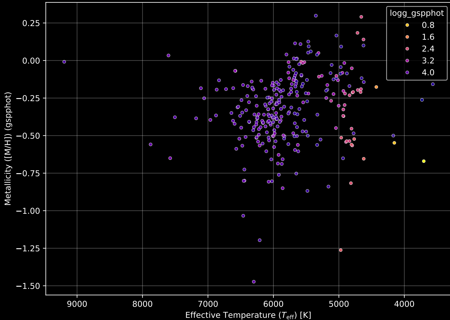
GALAH DR4 Field: [2547] Stellar Population Parameters (n= 276)
