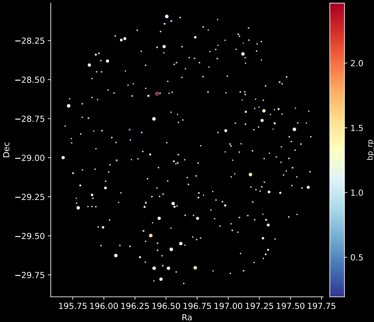
GALAH DR4 Field: [2547] Stars: 276
