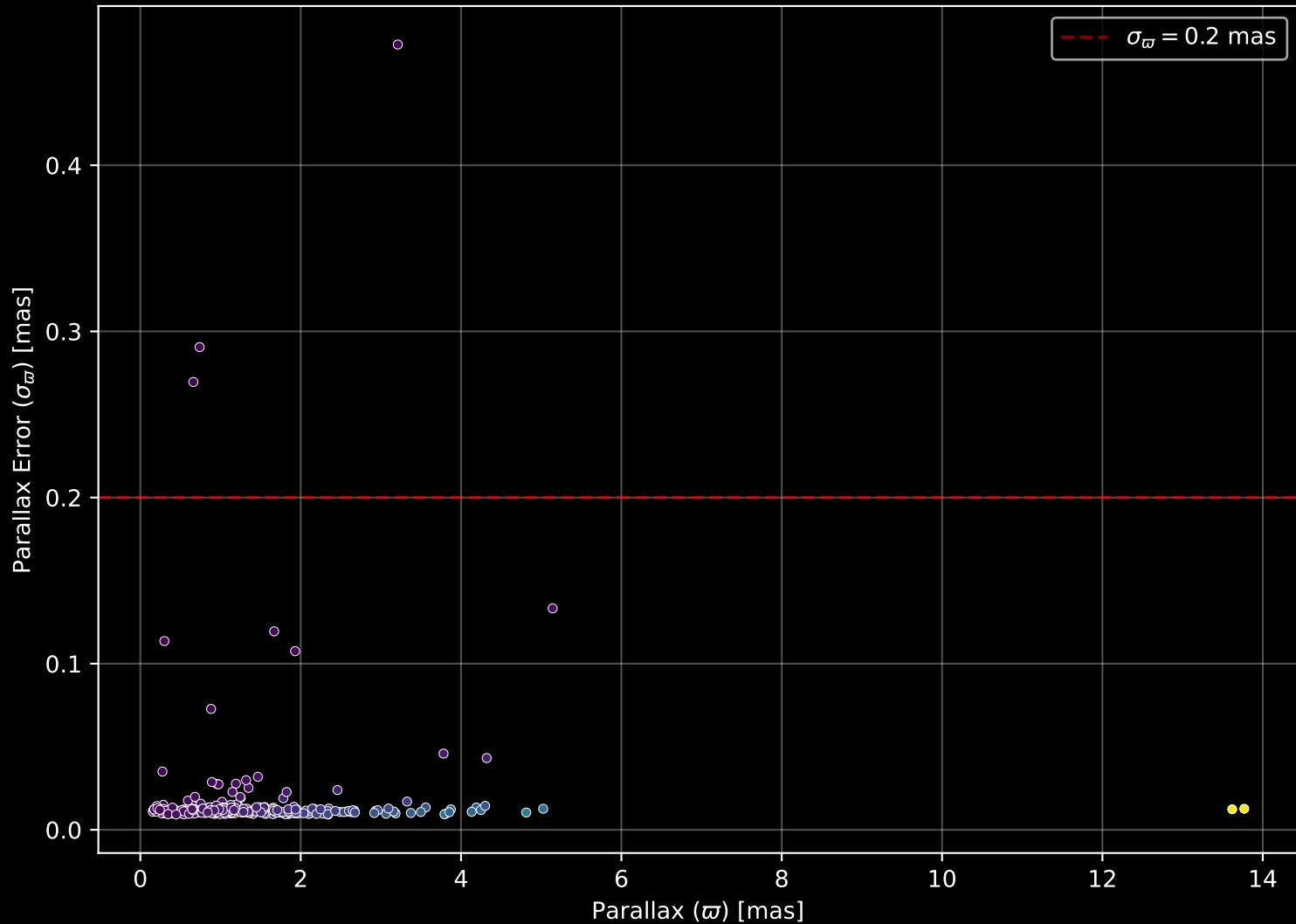
GALAH DR4 Field: [2547] Parallax Quality (n= 276)
